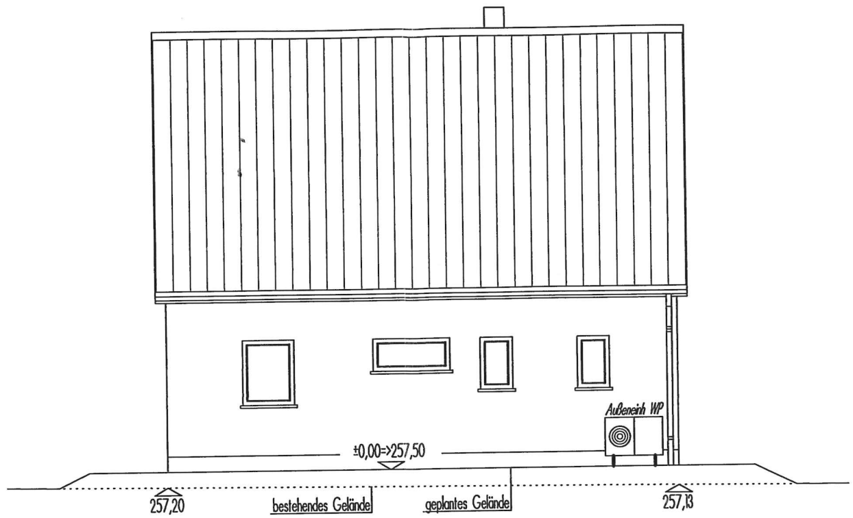
Nord Ansicht
